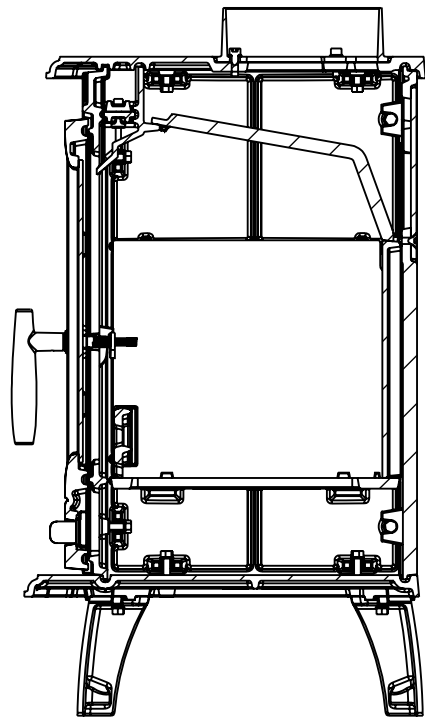
PRZEKRÓJ A-A
